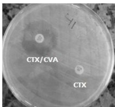
شکل ۱. ردیابی تولید آنزیم‌های بتالاکتاماز وسیع الطیف (ESBLs) به روش دیسک ترکیبی. CTX: سفوتاکسیم، CTX: سفوتاکسیم، CVA: کلوالانیک اسید.
