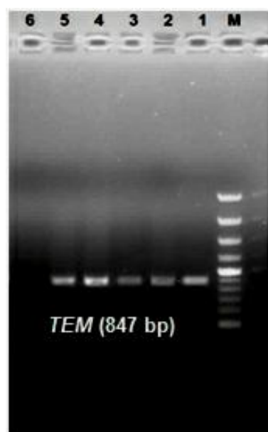
شکل ۲. آگارز ژل الکتروفورز محصولات PCR حاصل از تکثیر ژن TEM. M، DNA مارکر ۱۰۰ bp؛ ستون ۱، جدایه کنترل مثبت (واجد ژن TEM، اهدایی آقای دکتر ناظمی)؛ ستون‌های ۲ تا ۵، جدایه‌های /شریشی‌کلی مورد آزمایش حاوی ژن TEM؛ ستون ۶، سویه کنترل منفی (فاقد ژن TEM، ATCC 25922).
