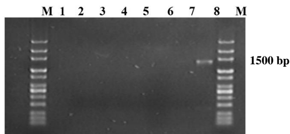
شکل ۳. PCR مربوط به ژن اینتگرون کلاس ۲. ستون ۱: کنترل منفی، ستون‌های ۲ تا ۷: نمونه‌های مورد مطالعه، ستون ۸: کنترل مثبت، M: مارکر وزن مولکولی.
