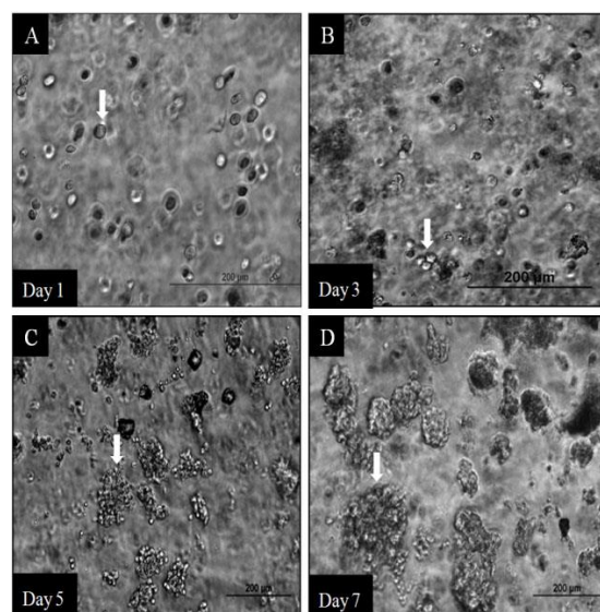
شکل ۳. بررسی فنوتیپ سلول‌های بنیادی عصبی قرار گرفته در هیدروژل پلی‌اتیلن‌گلیکول در روزهای ۱ (A)، ۳ (B)، ۵ (C) و ۷ (D). تجمعات سلولی با پیکان نمایش داده شده است.
