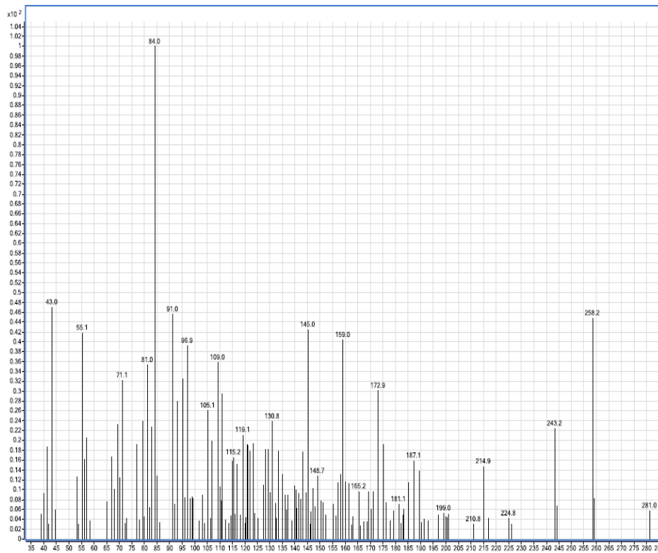
شکل ۱. کروماتوگرام حاصل از آنالیز GC/MS/MS اسانس برگ گیاه گزنه منطقه سه هزار تنکابن (محور افقی، نمودار زمان و محور عمودی، فراوانی است).
